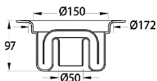
SIPHON VERTICAL DUSCHBRUNN - 090A
