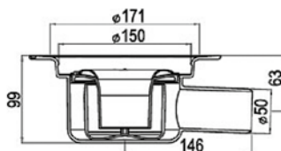
SIPHON HORIZONTAL FREJA - 090B
