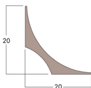
Forme d'appui (4011)
